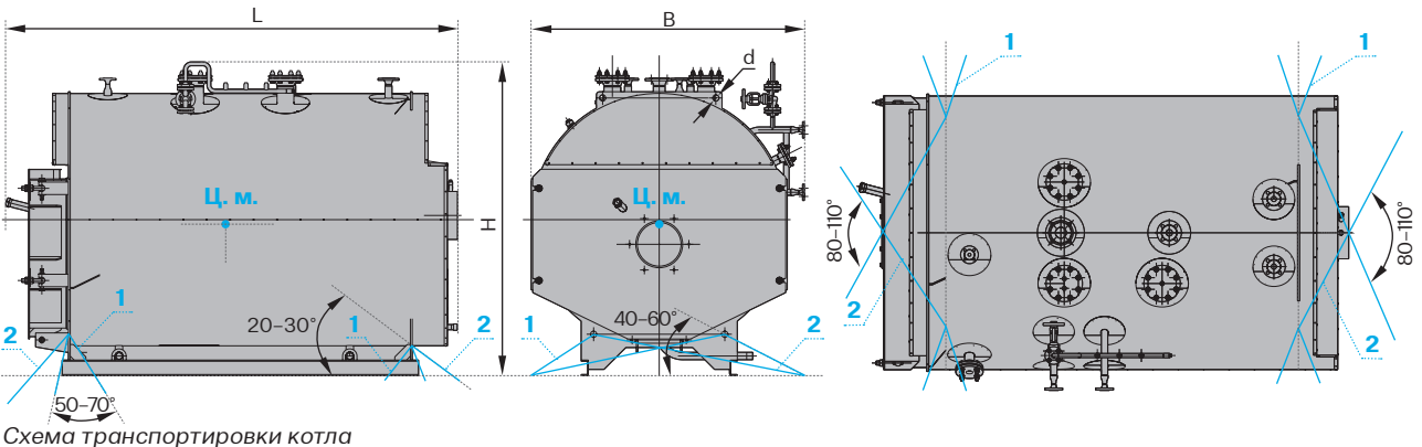
Схема транспортировки котла
